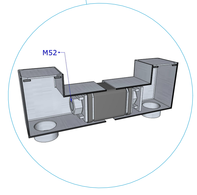
Laiturin liitososa Kumit joustavat aallokossa sallien ponttonien keskinäiset liikkeet. Pakkolukittu M52 kierreltiös. Kuormituksenkesto yli 80 tn (821 kN).
