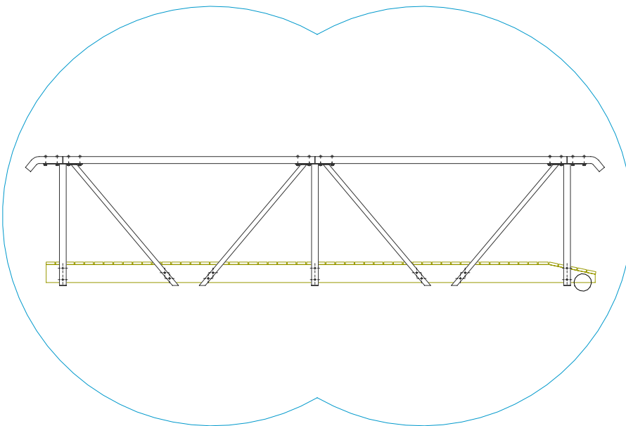
Jäykistävä teräskaide KS, 4,8-6 m käyntisillalle Pitkien käyntisillojen ja muiden pitkien jännevälien puurakenteiden jäykistämiseen ja käyttöturvallisuuden parantamiseen. Elementtirakenteinen, muokattavissa jälkikäteen. Kuumasinkittyä terästä.
