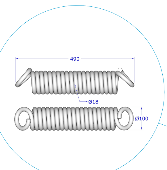
Teräsoustin 18 mm Raskasponttonilaitureiden rantakettingin jousin. Keventää kettinkien, kiinnikkeiden ja teräsoustimien kuormaa. Ottaa vastaan kettinkiin ja kiinnikkeisiin kohdistuvia voimia. Valmistettu sähkösinkitystä jousiteräksestä.
