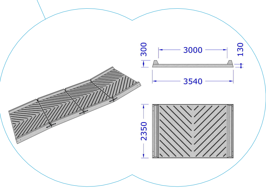
Venelaskuluiska 3 x 2,35 m Järeä, asennusvalmis betonielementti. Reunavahvistettu. Elementit kiinnitetään toisiinsa kuumasinkityillä nivellaatioilla. Reunakorokkeet estävät renkaiden luistamisen reunan yli. Pinnan uritus takaa hyvän pidon.
