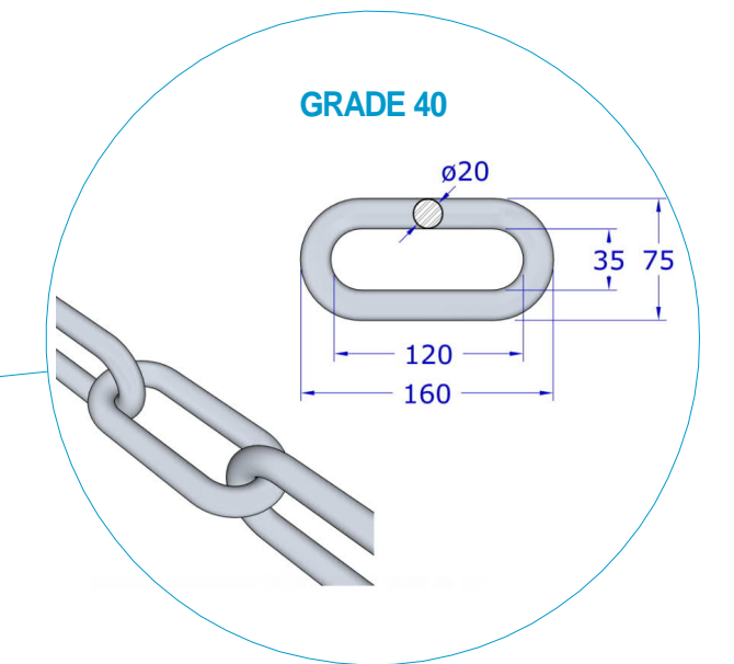
Kettinki pitkäahlo 20 mm, G40 / 15 m Grade 40 lujuustuokiteltu pitkäahlokettingi, jonka lujuusvaade on n.1,6 kertainen tavalliseen DIN763 kettinkiin verrattuna. Jokainen kettinki koekuormitettu. Kuumasinkitty (ISO1461). Paino 7,0 kg/m, työkuorma 4,1 tn, murtolujuus 25,6 tn
