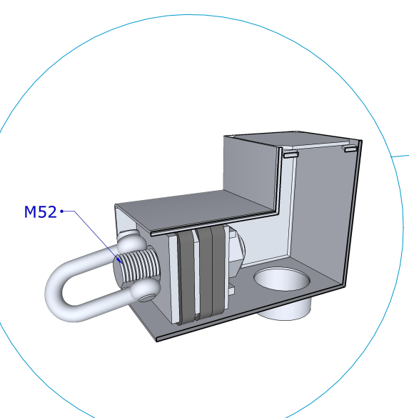
Laiturin ankkurointioustin kaivoon Joustava kiinnike raskasponttonilaitureiden rantakettingeihin. Kumirakenne ottaa vastaan kettinkiin kohdistuvia voimia. Keventää kettinkien, kiinnikkeiden ja teräsoustimien kuormaa. Järeä M52 kierreltiös. Pakkolukittu.
