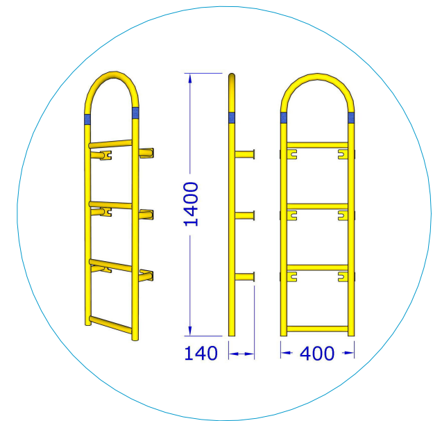
Turvatikas keltainen Merenkulkulaitoksen venesatamien turvallisuusohje edellyttää 25 m välein. Kuumasinkitty ja pulverimaalattu. Varustettu heijastimin.
