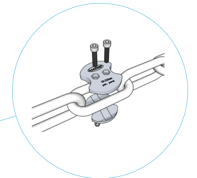
Kettinkisinkki 13-22 mm DIN763 -kettingeille. Suojaa korroosiolta ja pidentää kettinkien ikää. Asennettavissa myös jälkikäteen. Patentoitu
